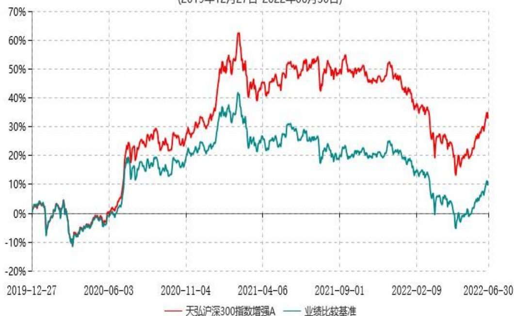
天弘沪深300指数增强A累计净值增长率与业绩比较基准收益率历史走势对比图
