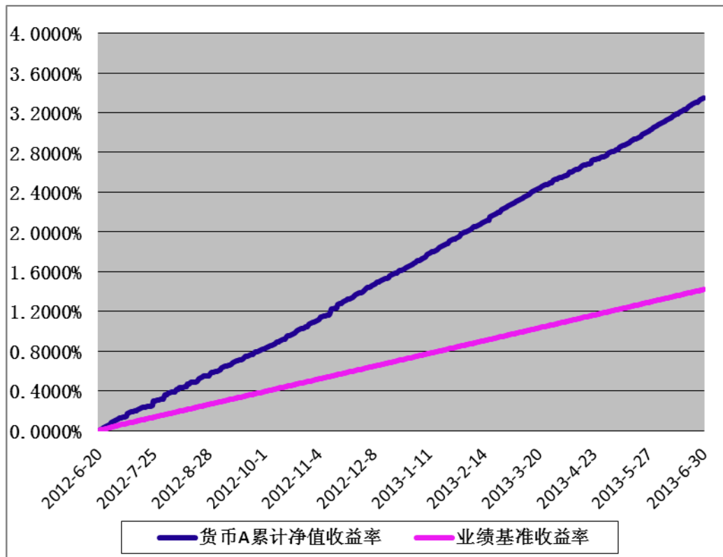
份额累计净值收益率与业绩比较基准收益率的历史走势对比图 (2012年6月20日至2013年6月30日)
